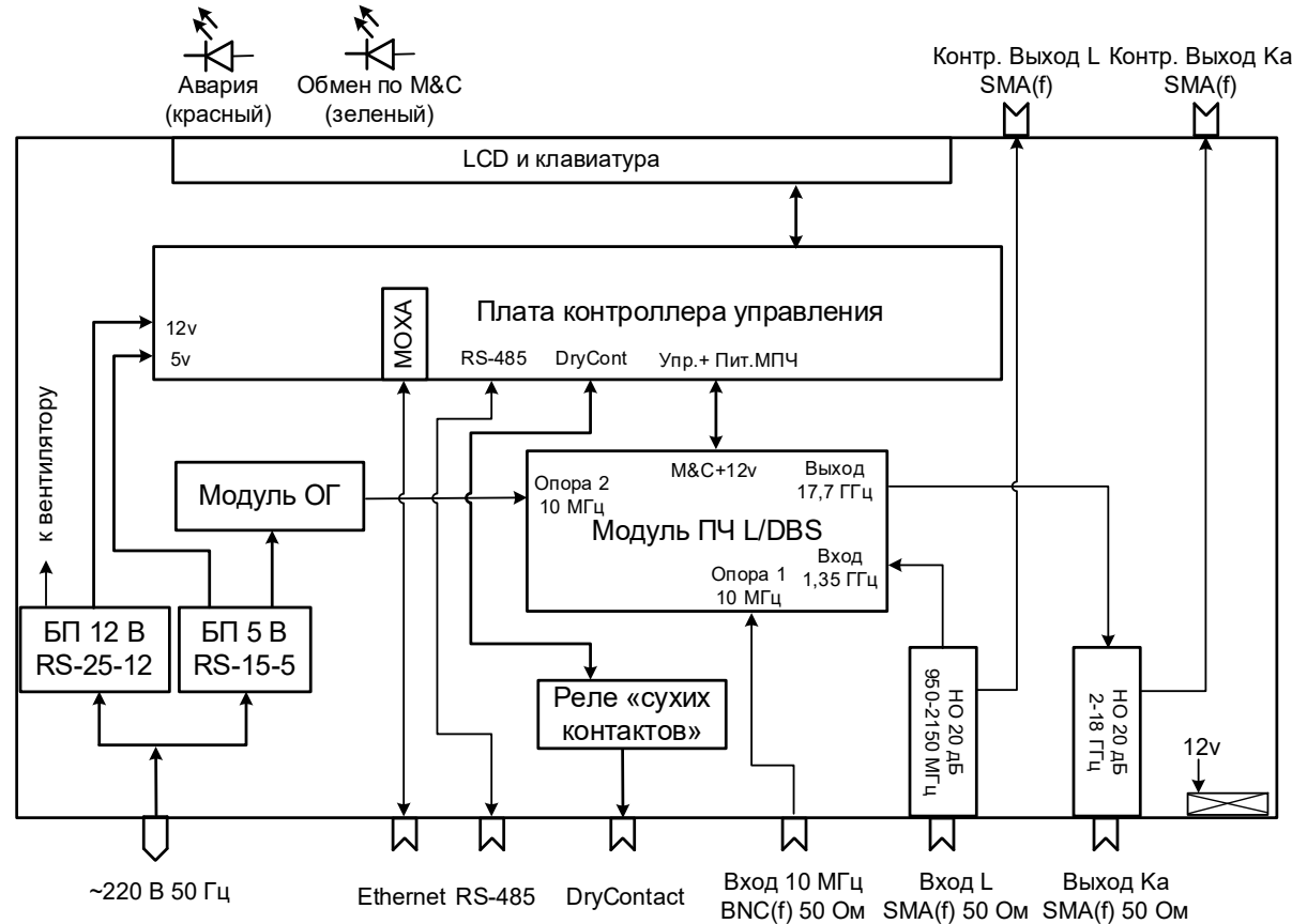
Рисунок 2 – Структурно-функциональная схема ПЧ «вверх»
